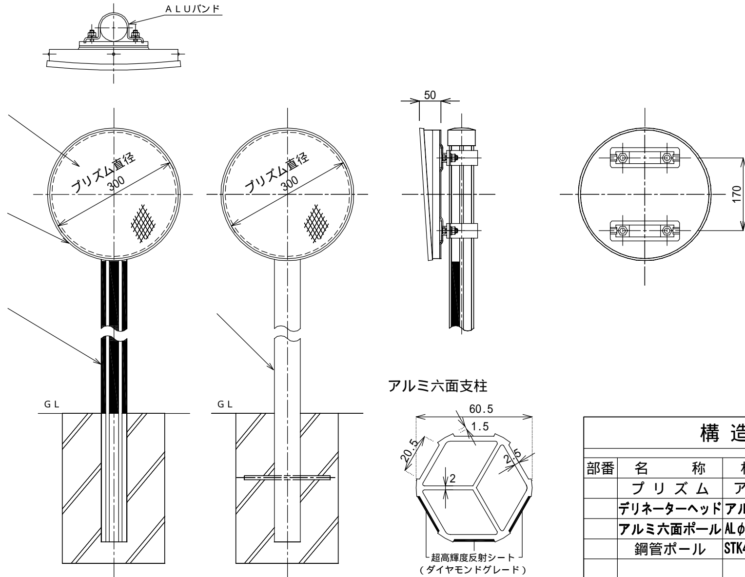
KD6300 - 型 (アルミ六面ポール) -超高輝度反射式-
