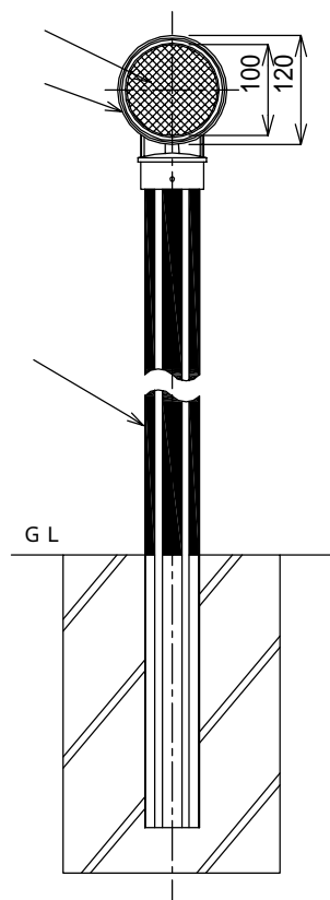
KD6100S - 型 (アルミ六面ポール) -超高輝度反射式-
